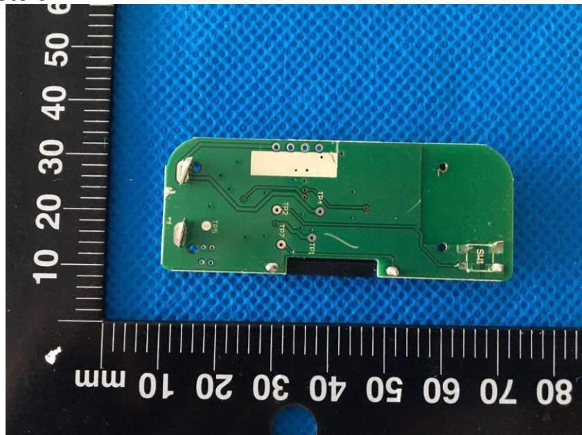
EUT Photo 6
