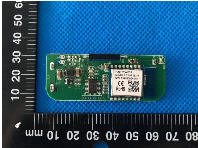
EUT Photo 5
